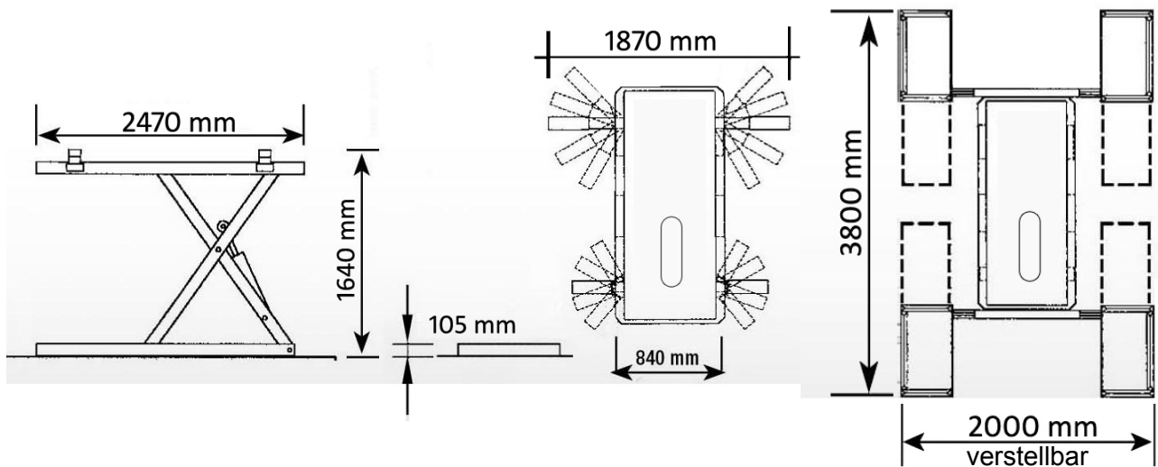
EH Elektrohydraulisch
